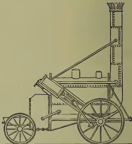
Fig. 2.—The 'Rocket.'
